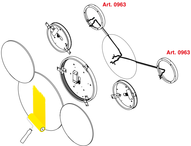
Esempio di installazione multipla con distanziali. Example of multiple installation with spacers.
