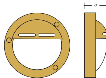
ART. 186.Gx53 ART. 186.G9 H. 5 - Prof. 5 - Ø 14 - G9 25 Watt
