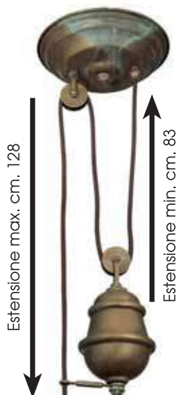
Art. 1354.T.AR (con vetro/with glass)
