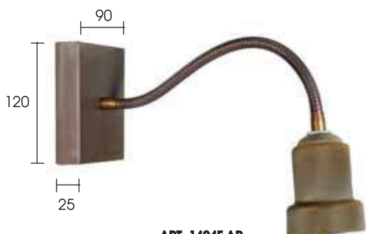
ART. 1424F.AR H. 120 - Larg. 300 Max Watt 28
