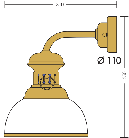
ART. 1008 Vetro Ø 250 - Larg. 250
