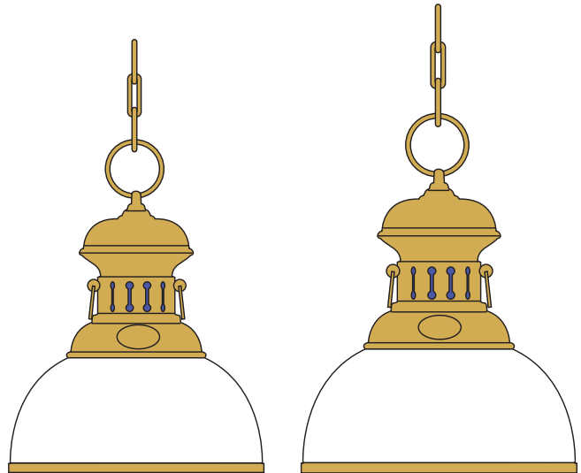
ART. 1010 Vetro Ø 250 - H. 370
